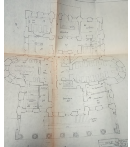
План I поверху палацу Кирила Розумовського, 1967 р., зібрання «УкрНДІпроектреставрація», фонд 166.
